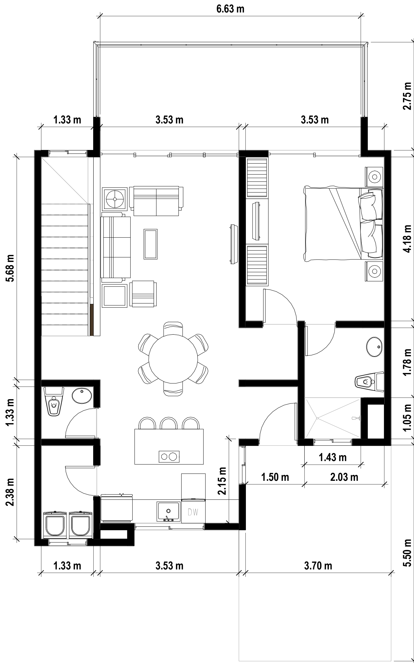
2 Level 1 ESCALA 1 : 50
